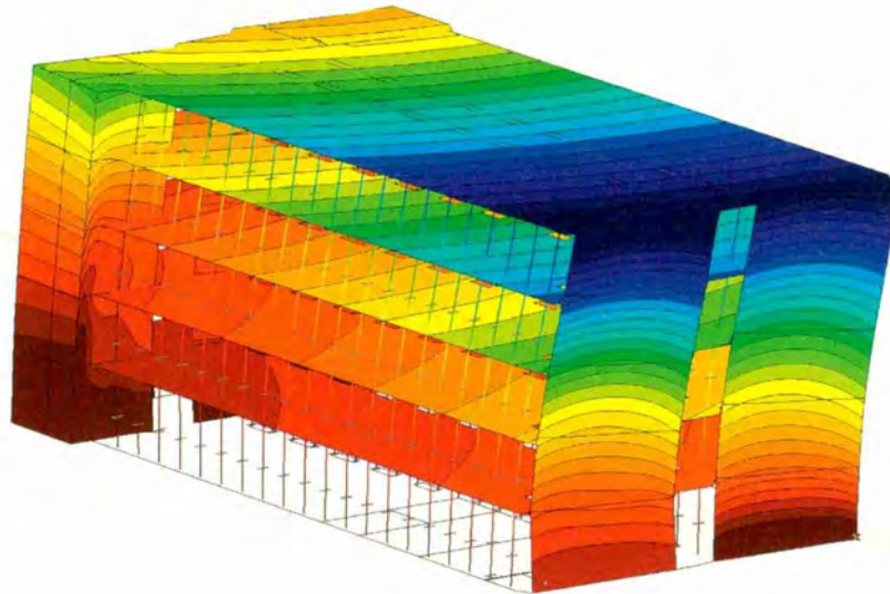
Auszeichnung: Kraft- und verformungsbasierte Erdbebenberechnungen als Grundlage für die Bemessung zweier Stahlbetonwände führen zum Erhalt eines Zürcher Laborgebäudes.
