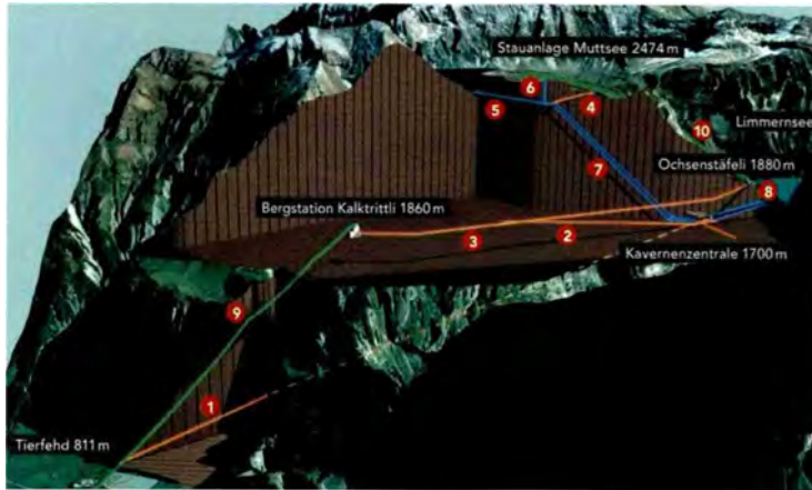
Übersicht über die Erweiterungsbauten beim Projekt Linthal 2015
