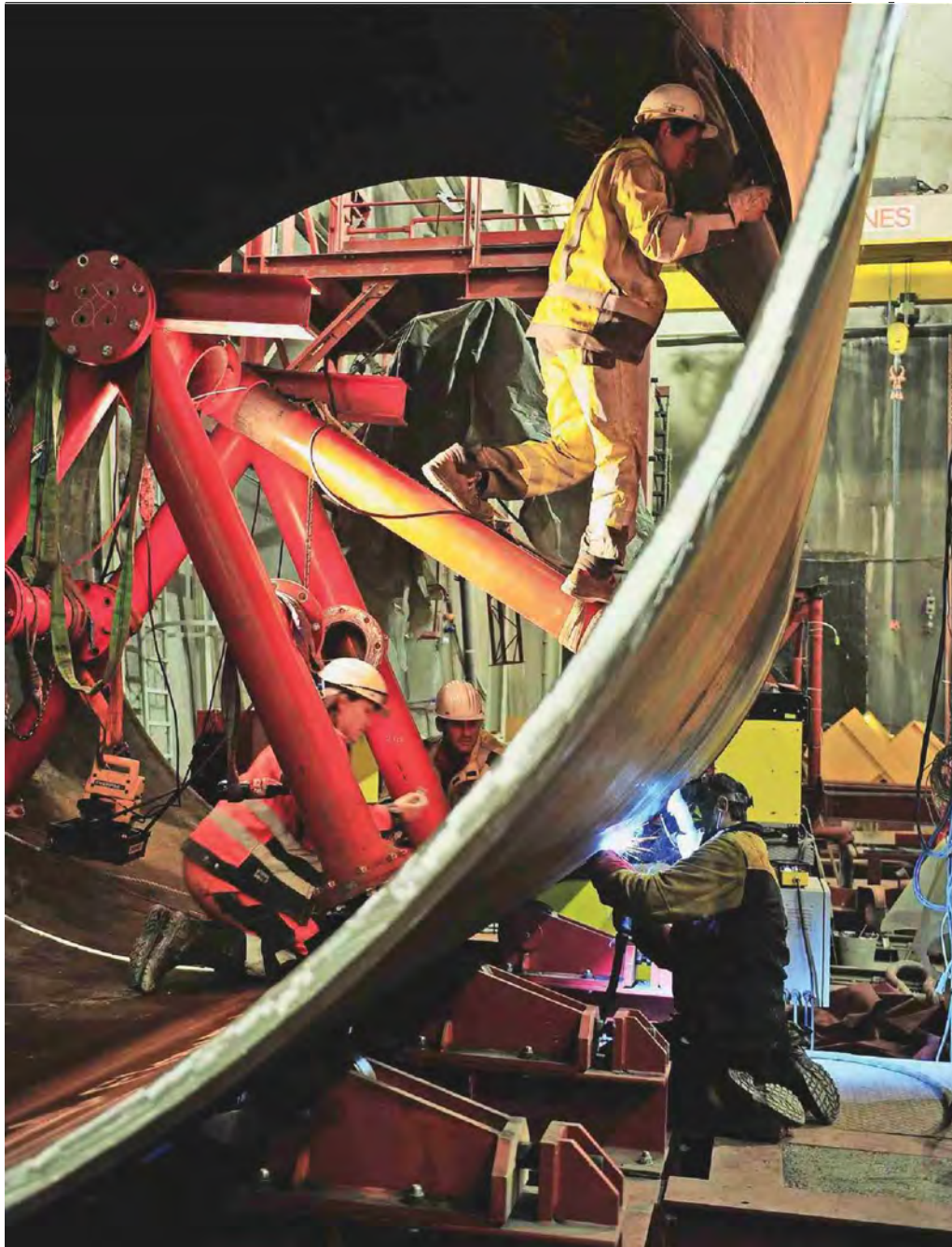
Im Wasserschloss Muttenalp wird das Druckrohr verschweisst und eingebaut
